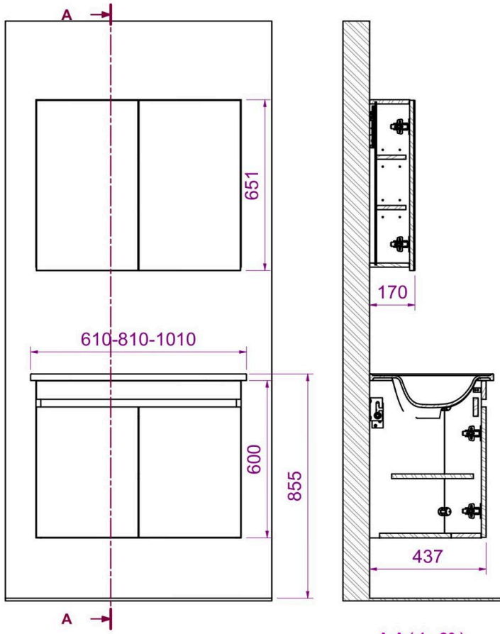
A-A (1 : 20)
